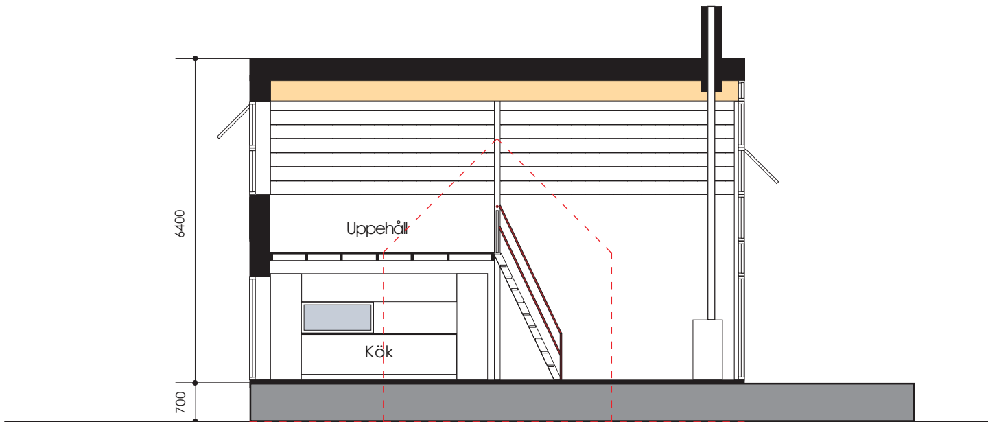
Sektion A/A
